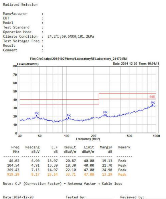
图 4-5 RE 测试水平方向
