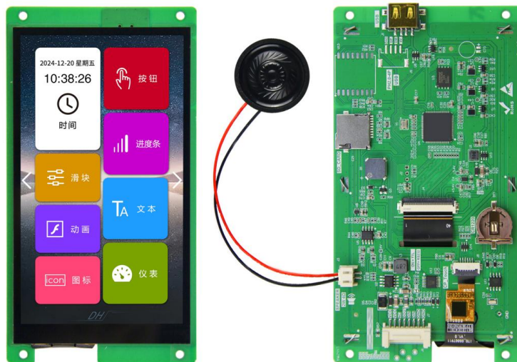
图 1-1 5.5 寸电容触摸参考图
